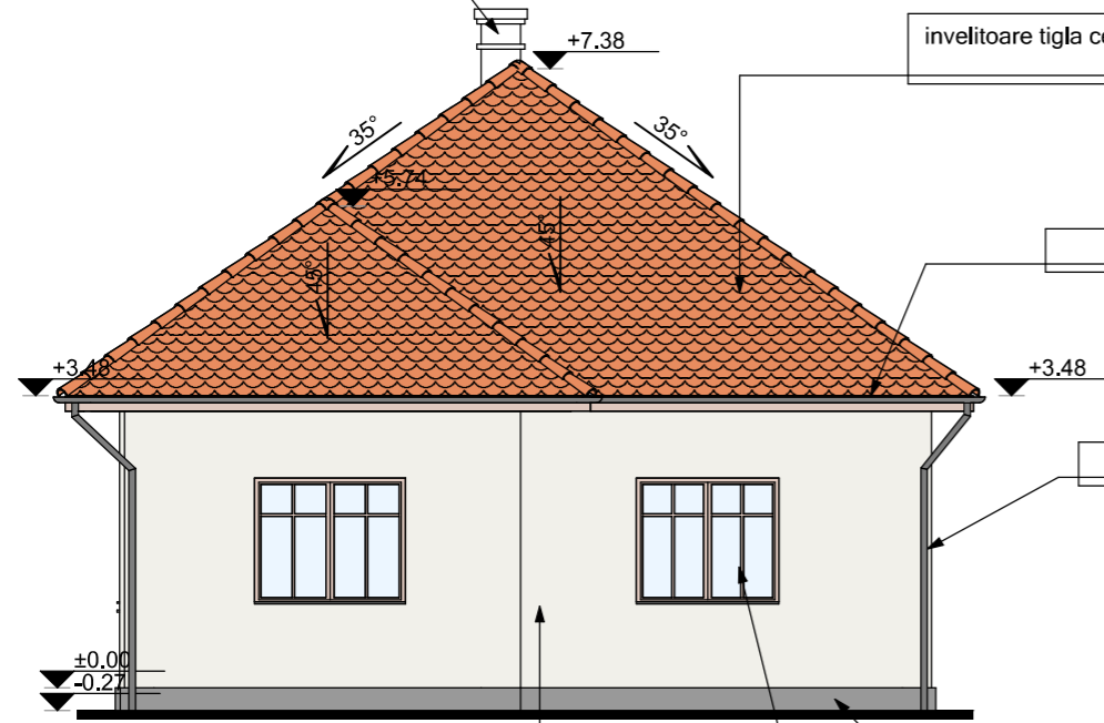
FATADA NORD SCARA 1:50
