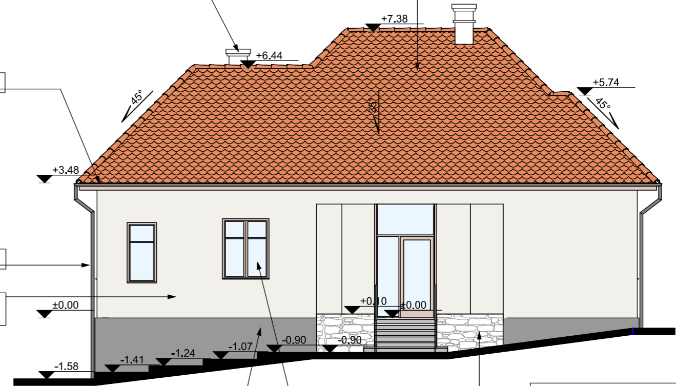
FATADA EST SCARA 1:50
