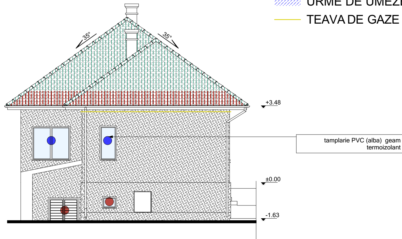
FATADA SUD SCARA 1:50
