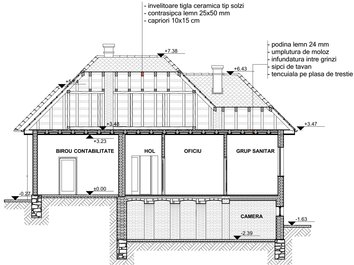
SECTIUNE A-A' SCARA 1:50
